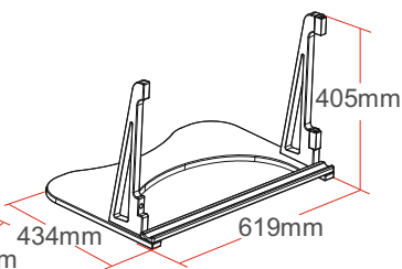
Standfuß (geneigt 5°)
