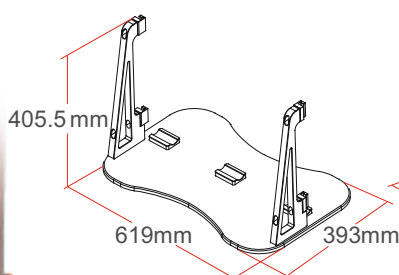
Standfuß (gerade)
