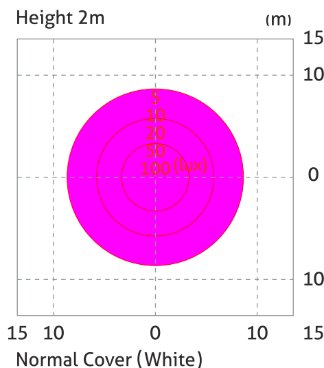
Polar Diagram (lux)
